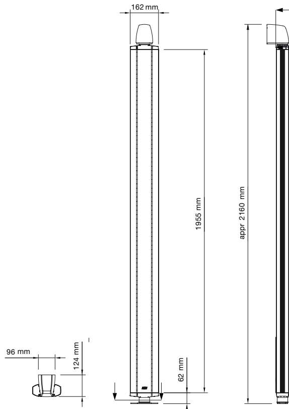
Steckdosenleiste auf der Rückseite montierbar.
